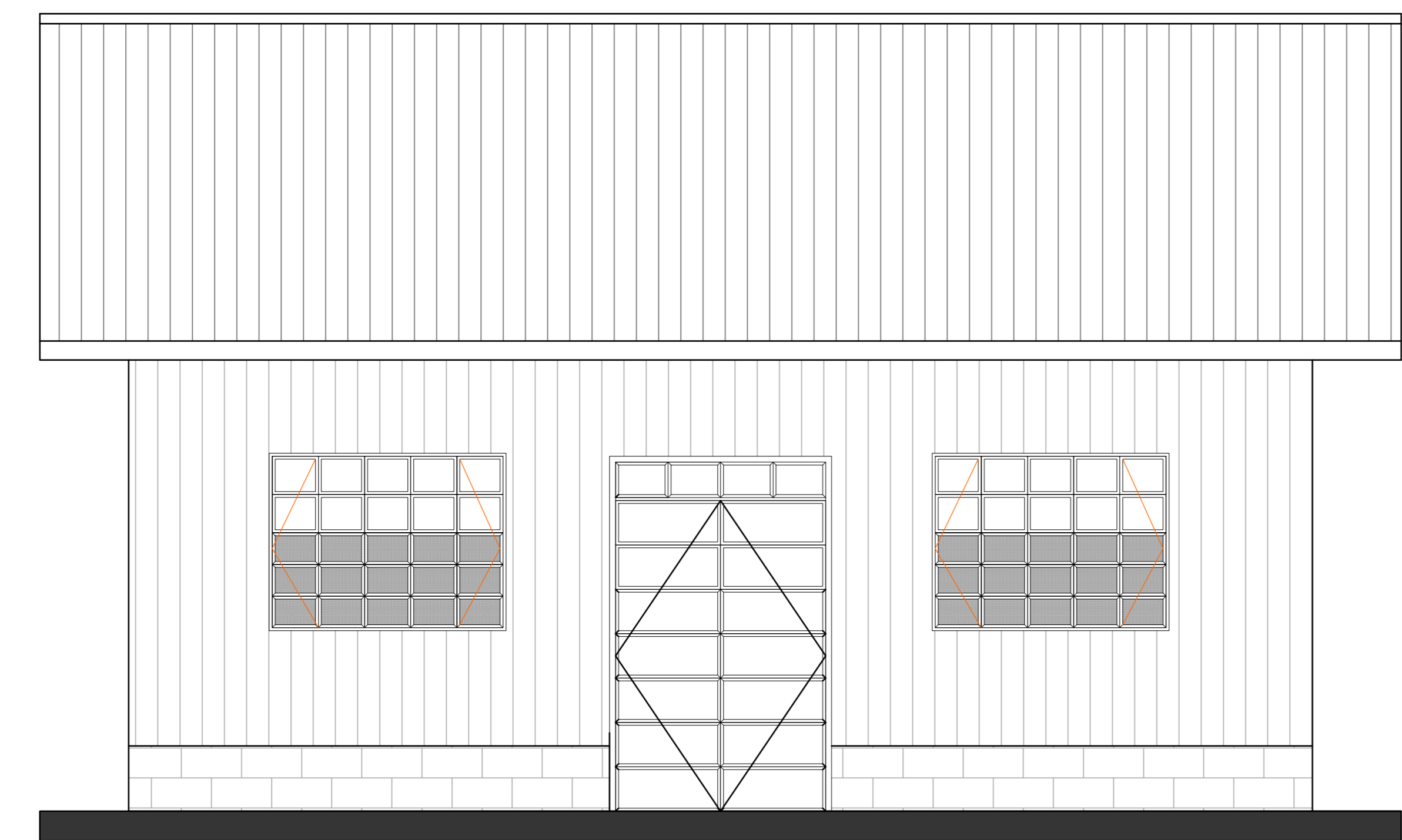
ELEVATION 02
